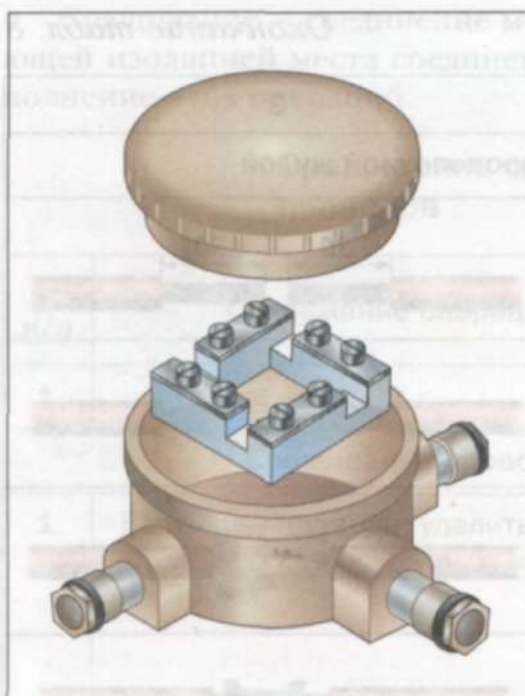
Рис. 30. Ответвительная коробка
