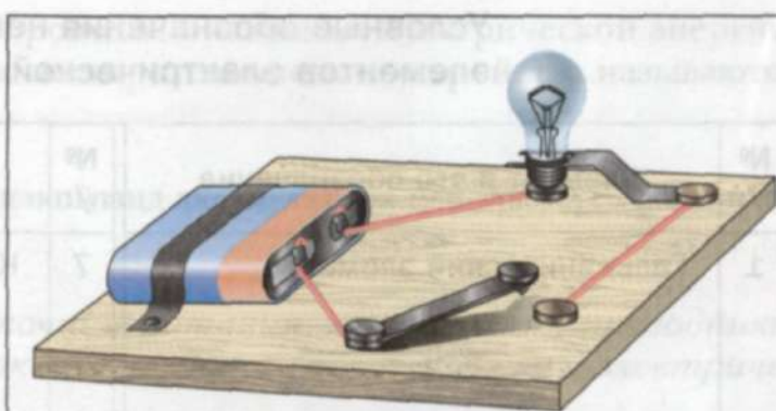
Рис. 18. Монтажная схема соединения элементов
