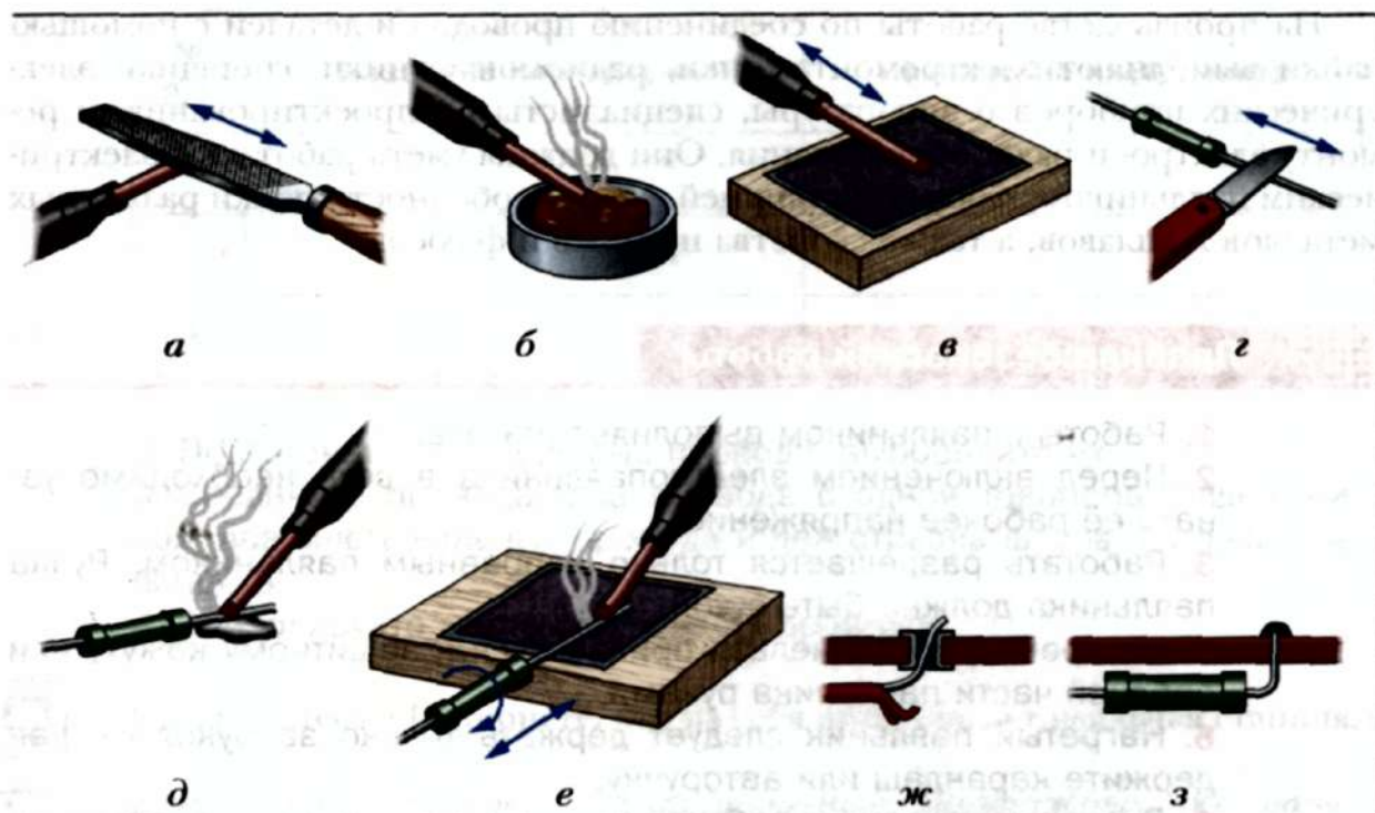
Рис. 34. Процесс паяния:
